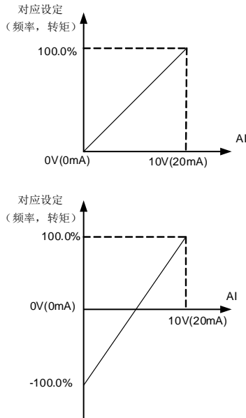
图 6-10 模拟给定与设定量的对应关系
