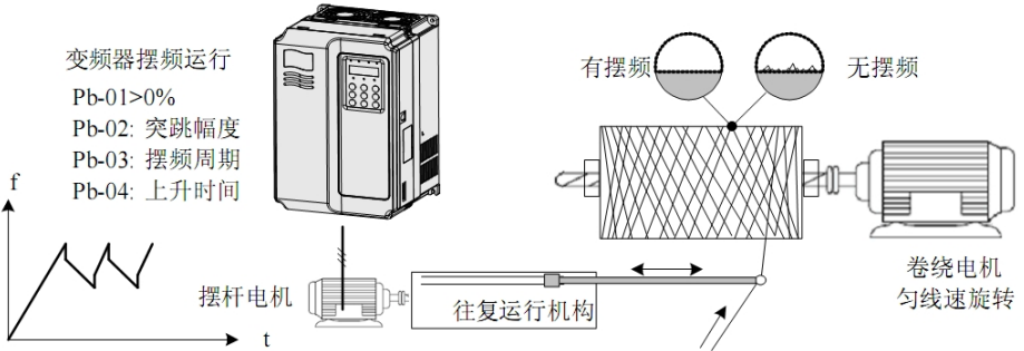
图 4-23 摆频工作模式
