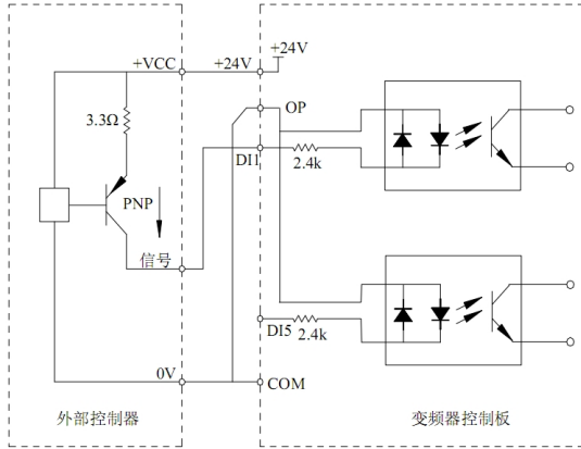
图 3-8 源型接线方式
