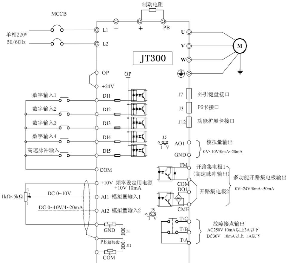
图 3-2 三相 380V/480V 变频器接线示意图
