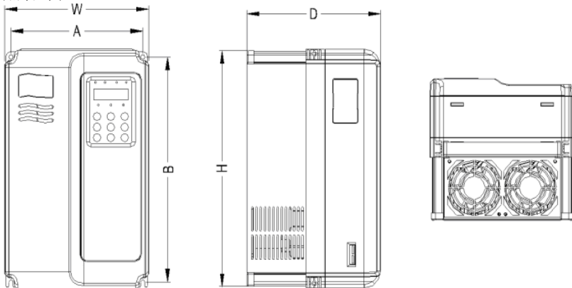
图 2-4 JT300 系列塑胶结构外型尺寸及安装尺寸示意图
