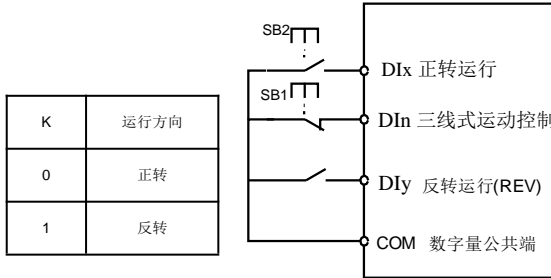
图 6-9 三线式控制模式 2
