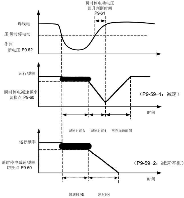
图 6-24 瞬时停电动作示意图
