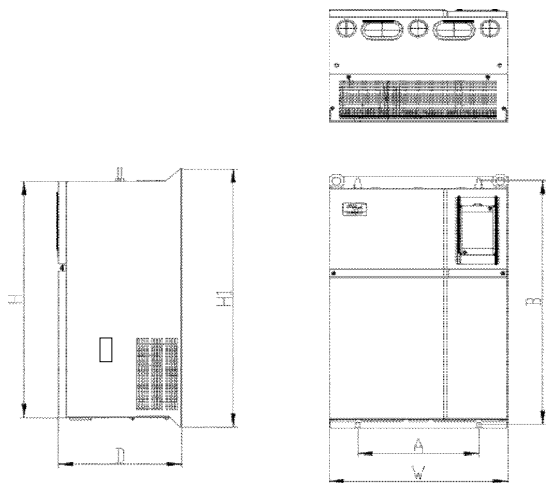
图 2-5 JT300 系列钣金结构外型尺寸及安装尺寸示意图
