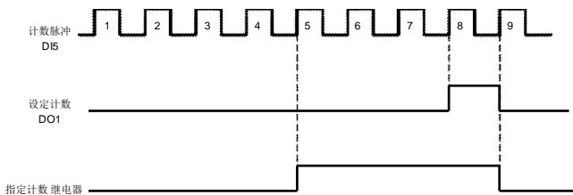
图 6-29 设定计数值给定和指定计数值给定示意图
