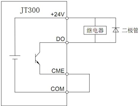
图 3-9 数字输出端子接线示意图
