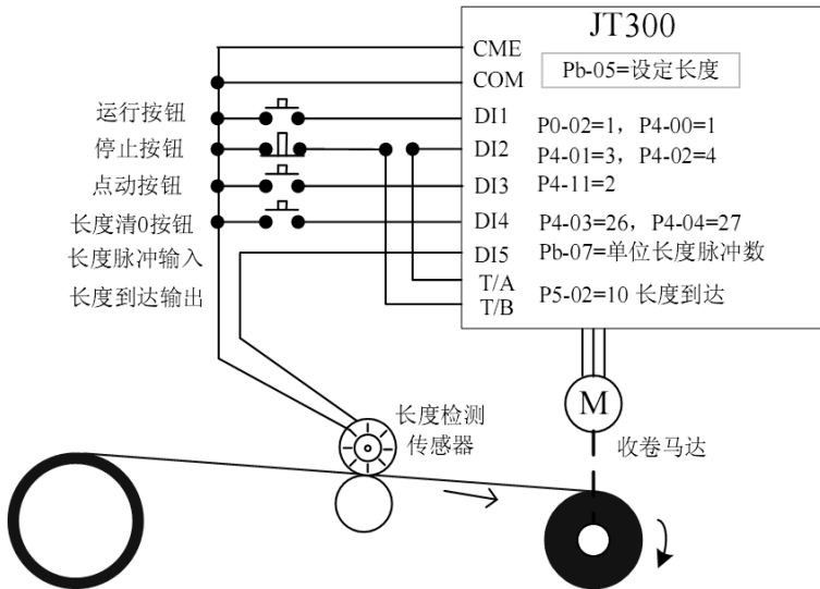
图 4-27 定长控制功能常见应用举例
