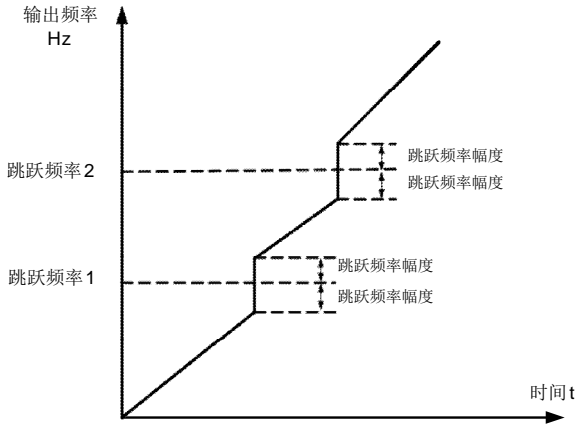
图 6-18 加减速过程中跳跃频率有效示意图
