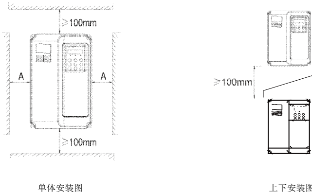
图 3-1JT300 变频器安装示意图
