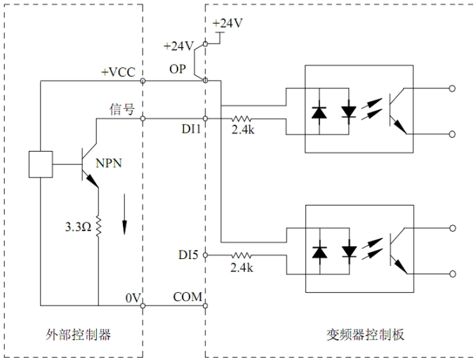
图 3-6 漏型接线方式
