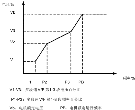
图 6-4 多点 V/F 曲线设定示意图
