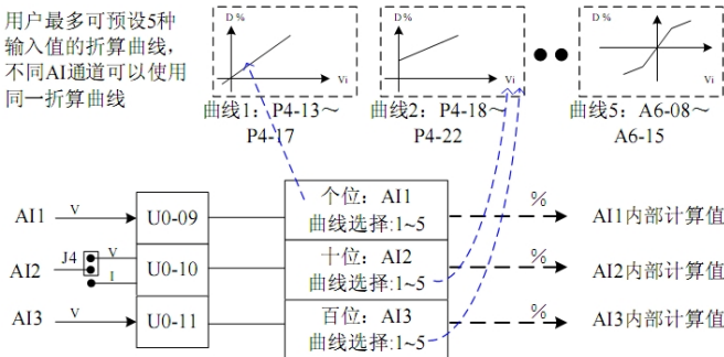
图 4-30 AI 信号对应实际给定
