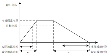
图 6-5 VF 分离示意图
