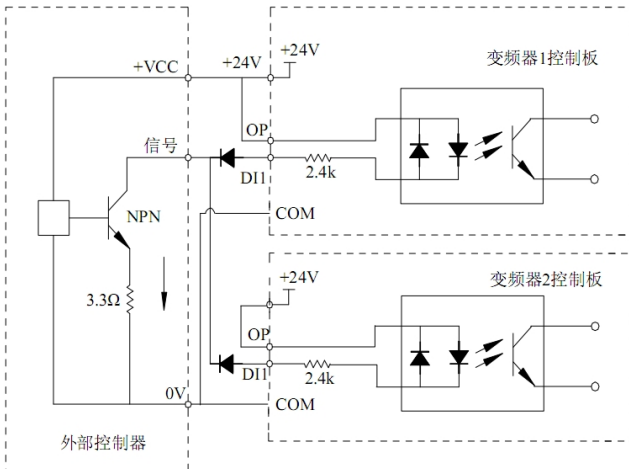
图 3-7 多台变频器数字输入端子并接漏型接线方式
